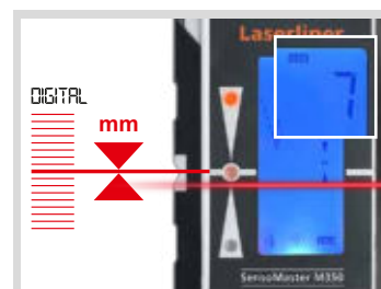
Indicazione al millimetro del dislivello dal piano laser
