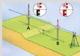
Scala visiva a distanza con graduazione E
