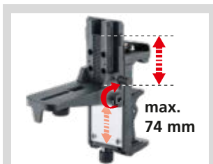
CrossGrip Pro Regolazione precisa
